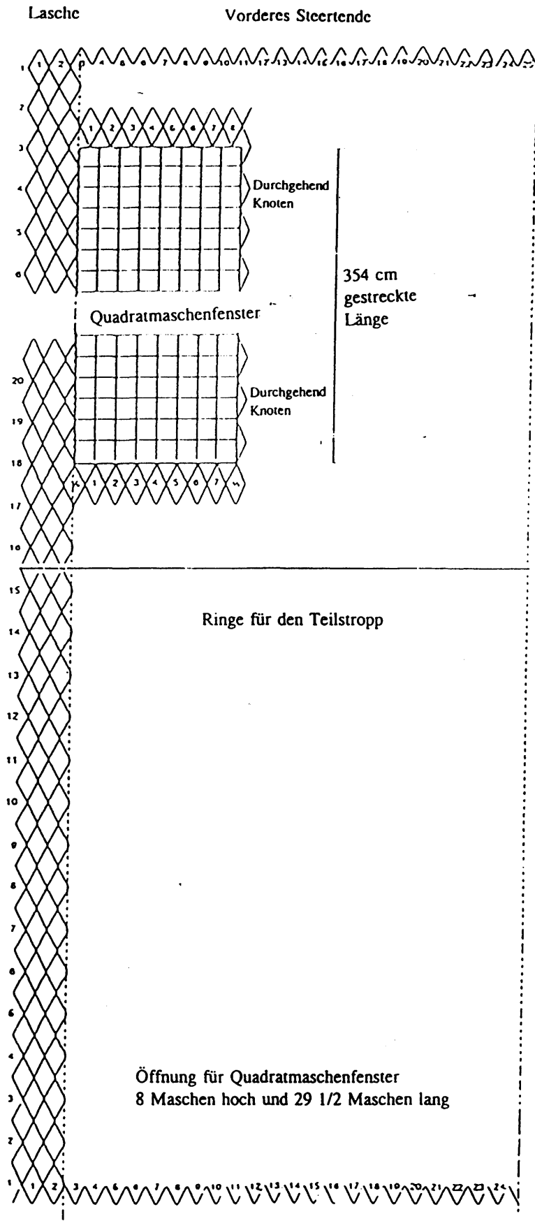
Schaubild 3: Einfügung des Fensters in den Steert Technische Beschreibung (Vorschlag)
