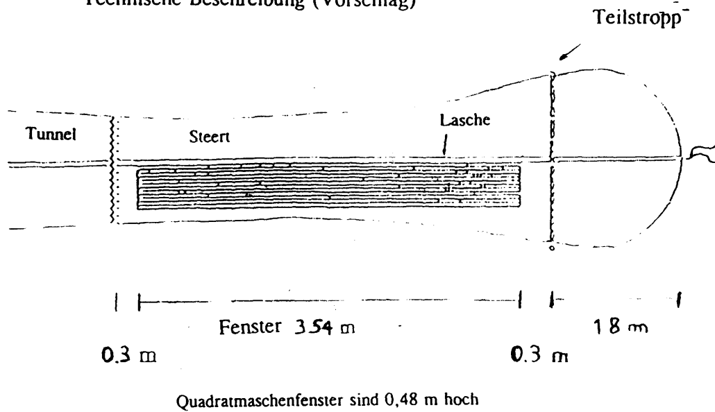
Schaubild 1: Anbringung der Quadratmaschenfenster im Steert Technische Beschreibung (Vorschlag)
