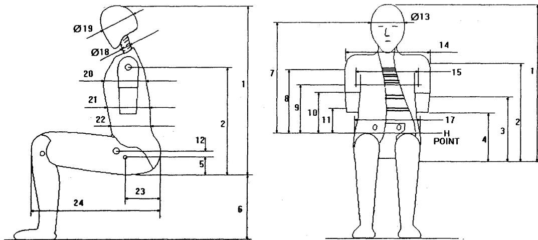
Abbildung 2 - Hauptabmessungen der Prüfpuppe
