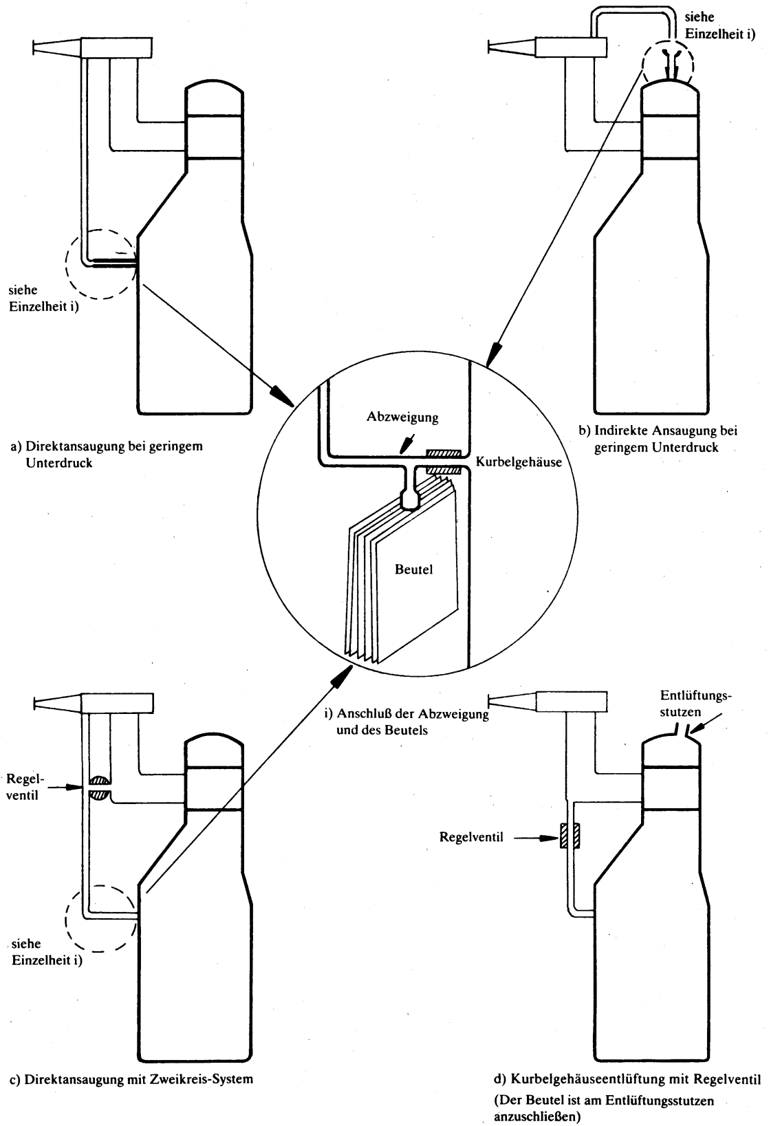
Abbildung V.5 Prüfung Typ III
