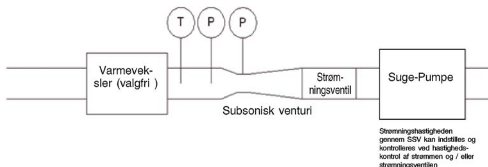
Skematisk tegning af et subsonisk venturirør (SSV)
