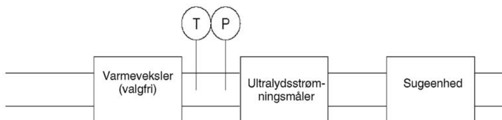
Skematisk skitse af ultrasonisk flowmeter (UFM)
