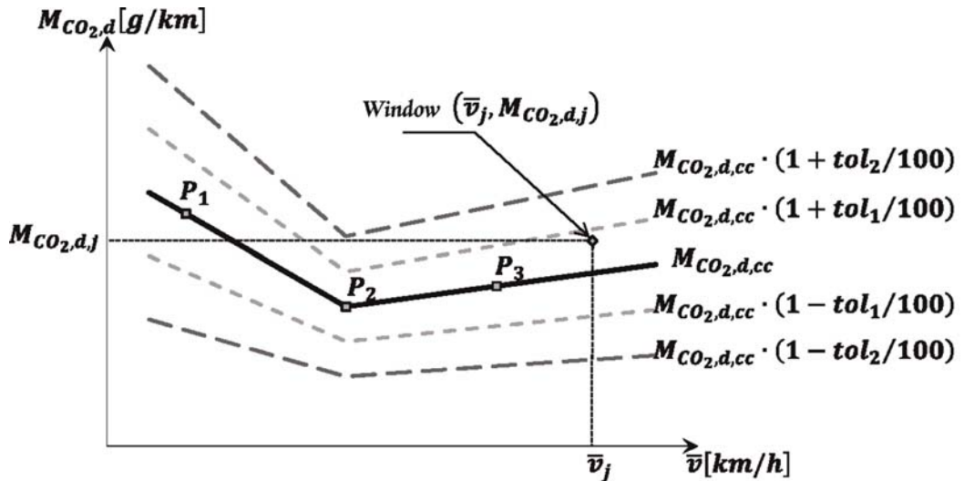
Køretøjets CO 2 -karakteristikkurve
