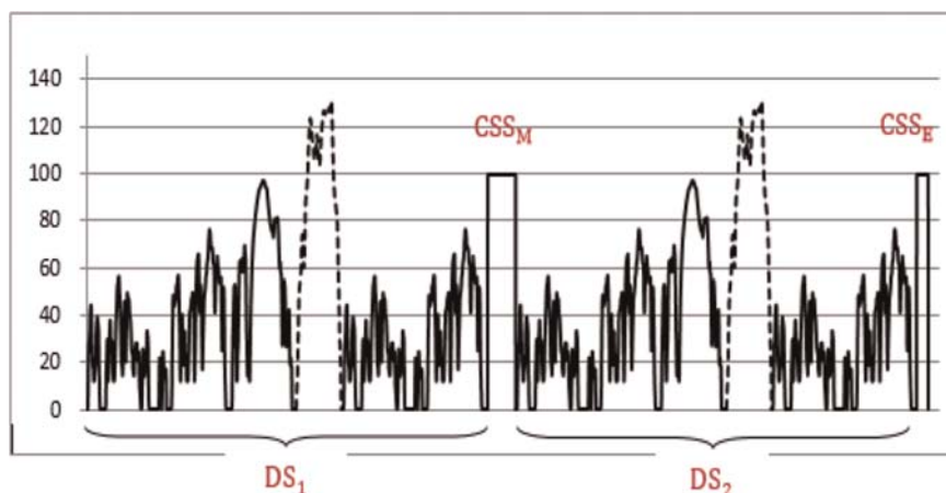
Hastighedskurve for forkortet type 1-prøvningsprocedure
