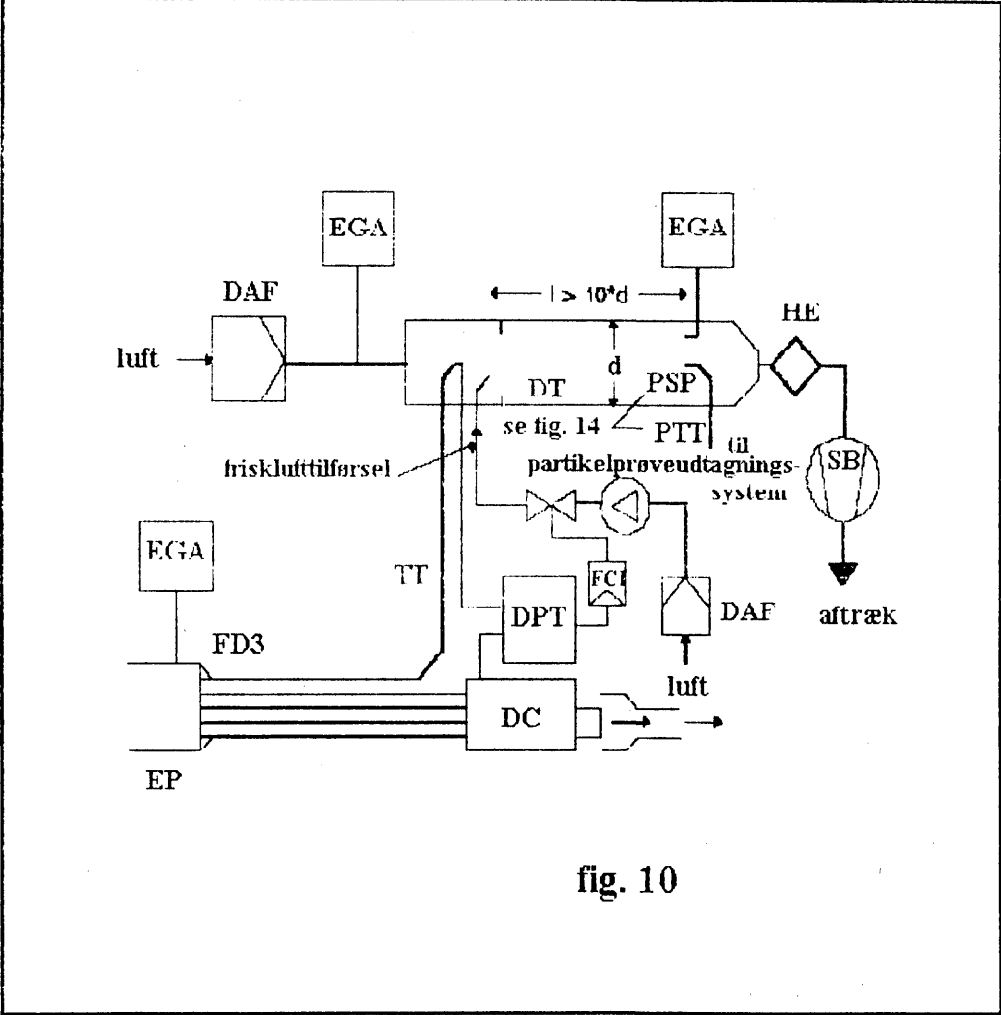
Fig. 10 Delstrømfortyndningssystem med forgrenede rør, koncentrationsmåling og delstrømprøveudtagning
