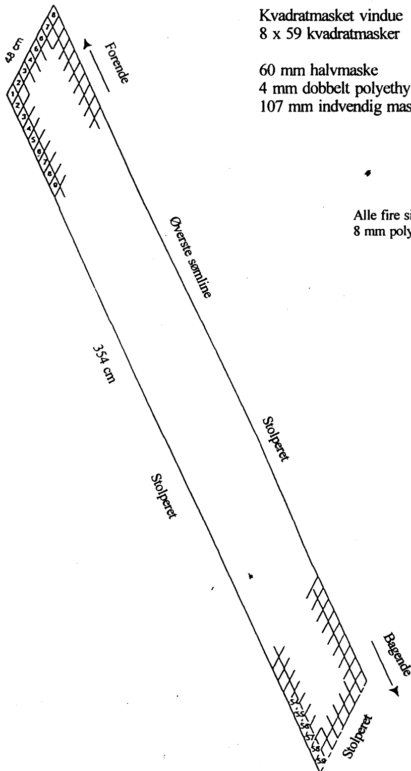
Figur 2 Netstykke til kvadratmasket vindue Forslag til specifikation
