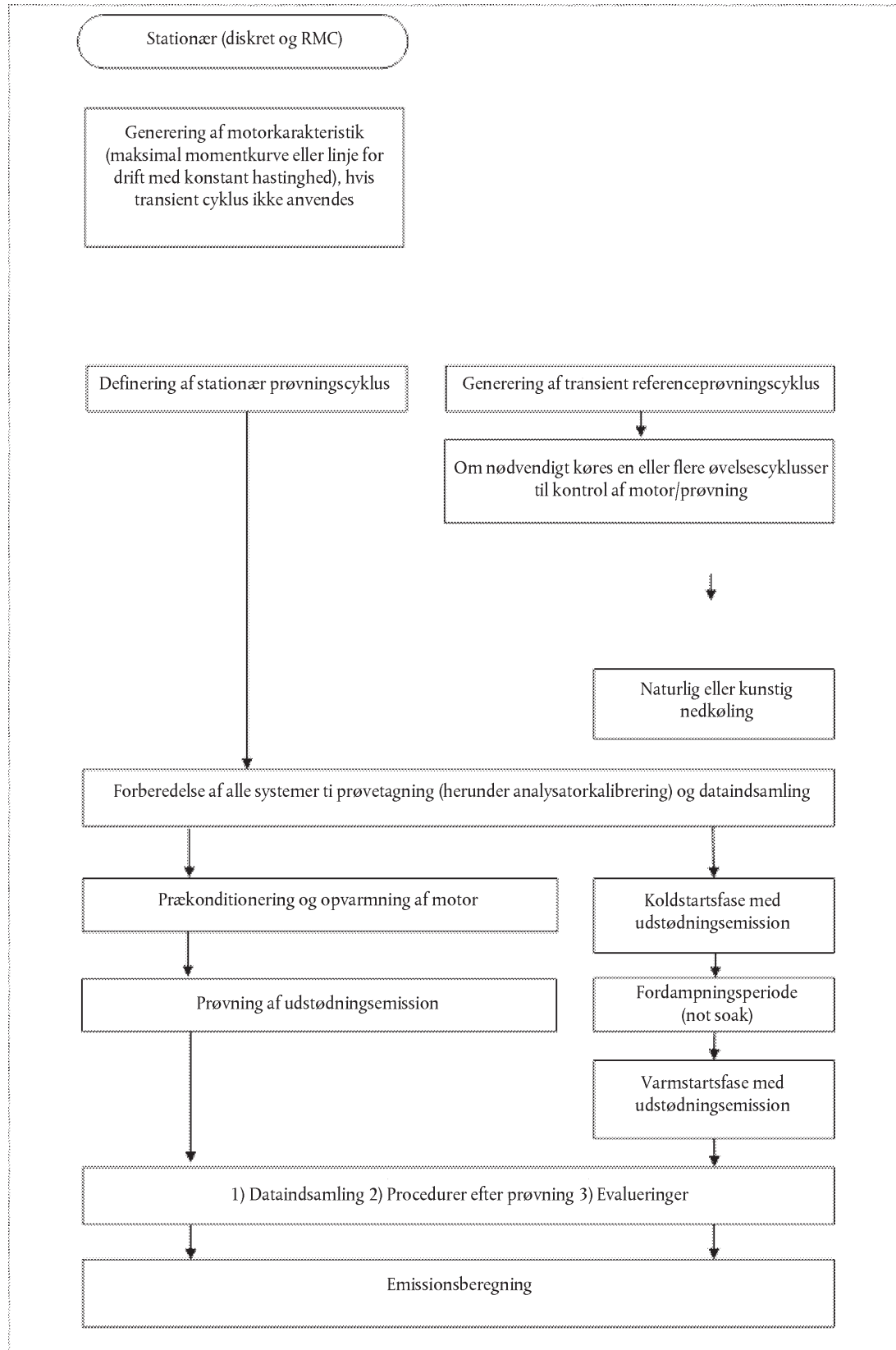
Figur 6.4 Prøvningssekvens
