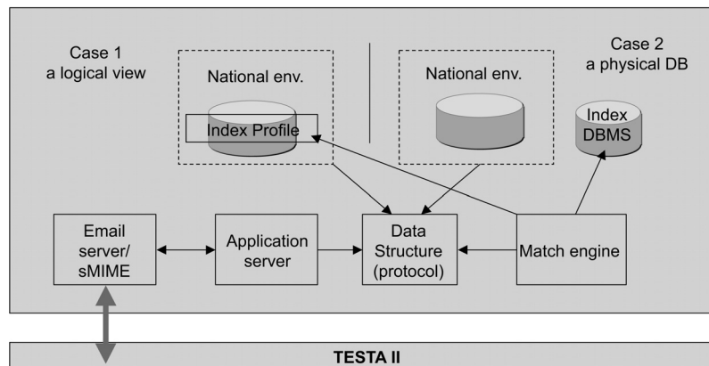
Figur 2: Skematisk oversigt over programmet
