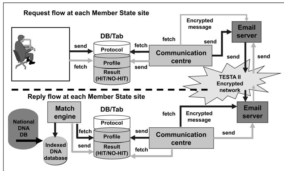
Figur 3: Oversigt over arbejdsgangen i databehandlingen på den enkelte medlemsstats operationssted
