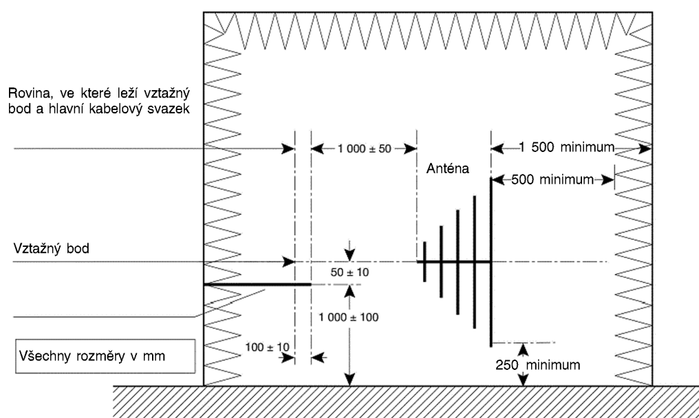
Pohled na rovinu podélné souměrnosti zkušebního stavu
