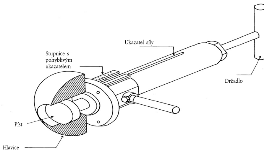
Obrázek 3 Zařízení k měření výčnělků
