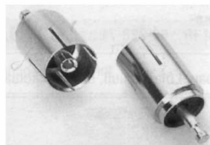
Obrázek 4 Koaxiální zásuvka
