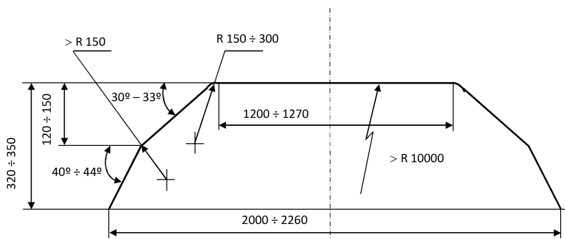
Obr.: Konfigurace a rozměry smykadel
