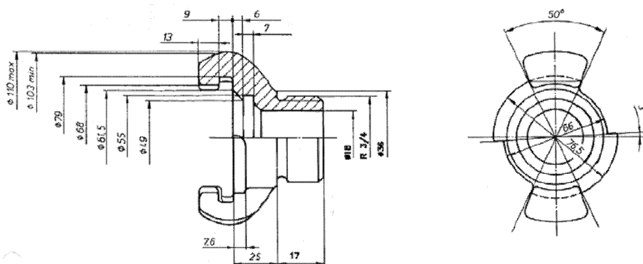
Obrázek A III Adaptér pro doplňování vody
