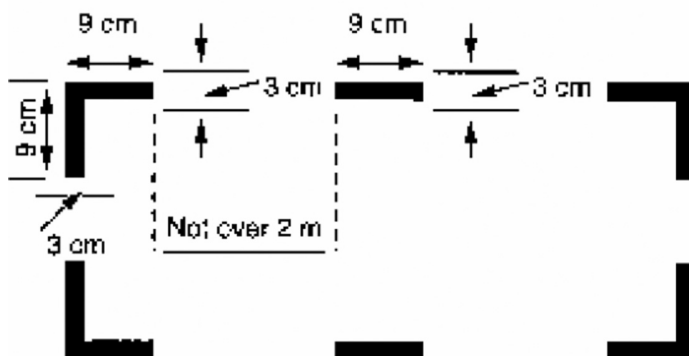
Označení míst pro vniknutí do trupu vrtulníku
