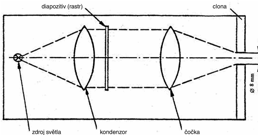
Obrázek 7 — Optické uspořádání promítacího zařízení
