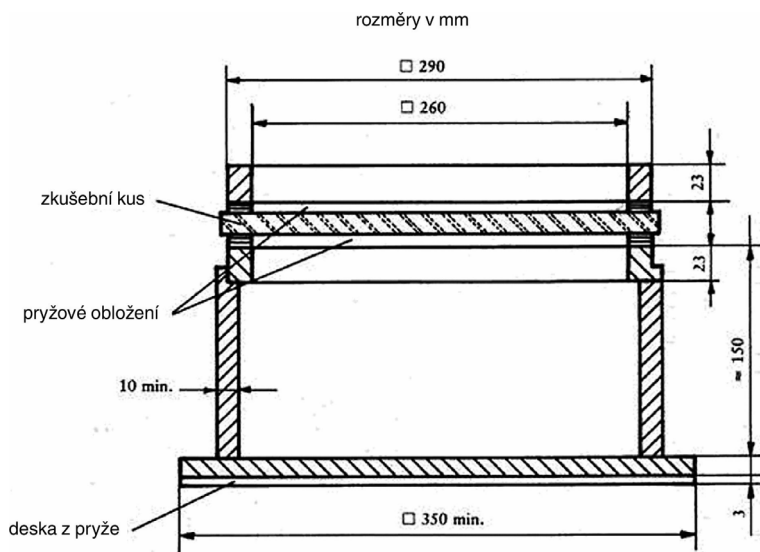
Obrázek 1 — Nosný přípravek pro zkoušky nárazem koule
