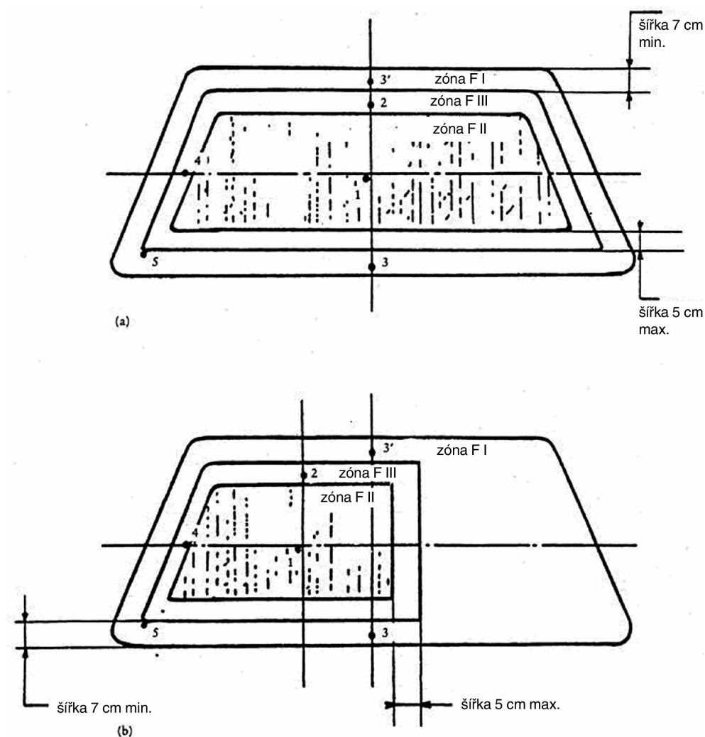
Obrázek 2 — Předepsané body nárazu pro tabule čelních skel
