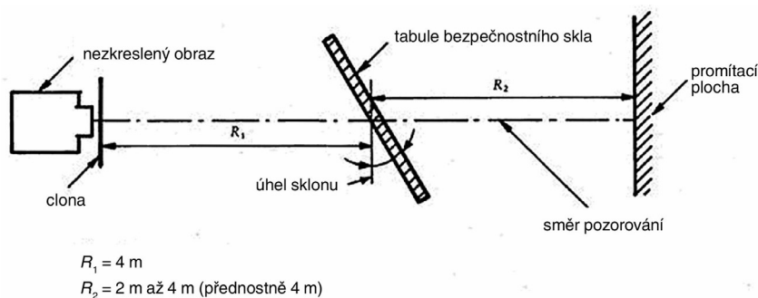
Obrázek 9 — Uspořádání přístroje pro zkoušku optického zkreslení
