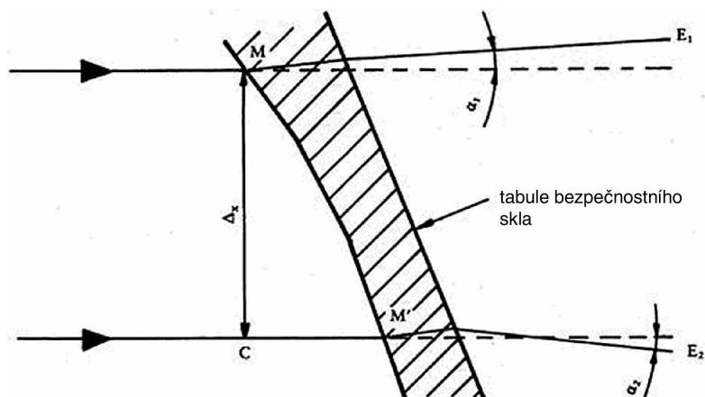
Obrázek 6 — Schematické znázornění optického zkreslení
