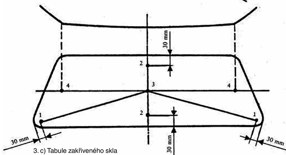
Obrázky 3a, 3b a 3c — Předepsané body nárazu pro tabule rovnoměrně tvrzeného skla
