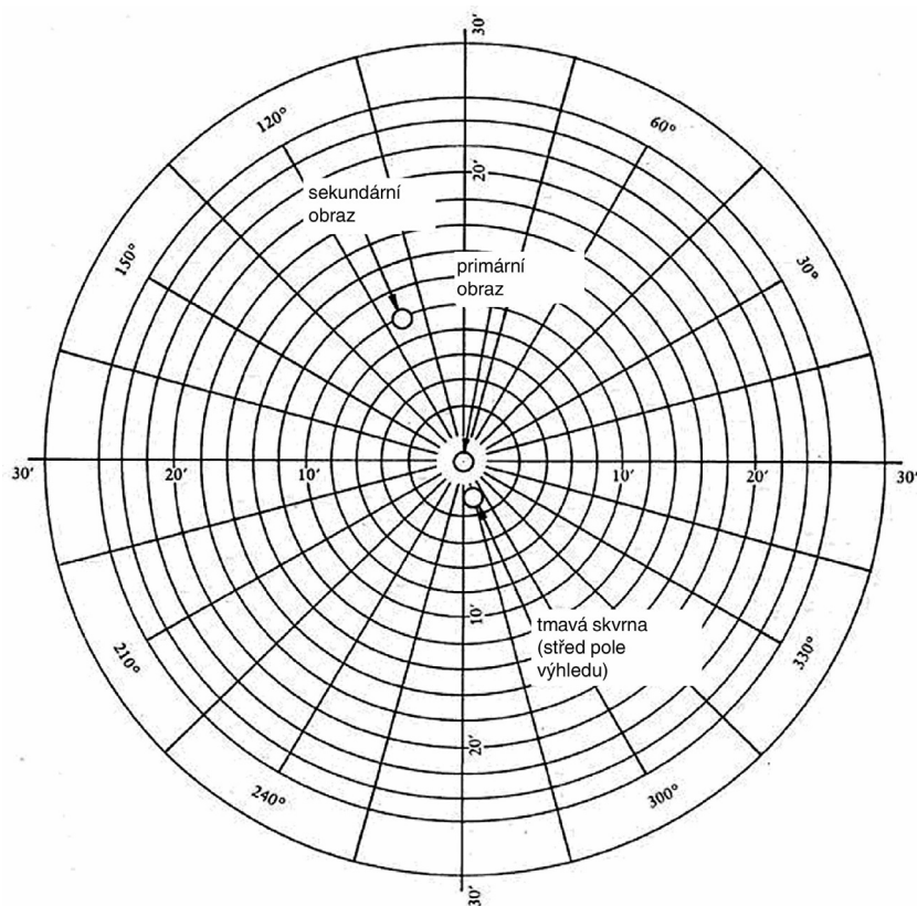
Obrázek 14 — Příklad pozorování při zkoušce s kolimačním dalekohledem
