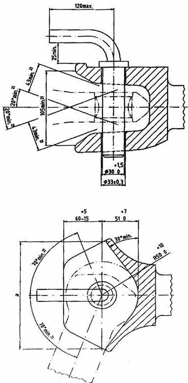
Obrázek 1a — Nesamočinné spojovací zařízení pro přívěs s válcovým blokovacím čepem
