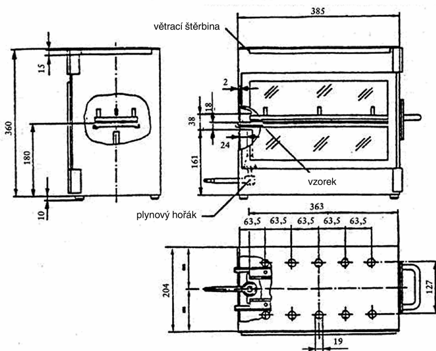
Obrázek 16 — Příklad spalovací komory
