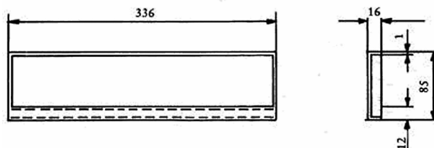
Obrázek 17 — Typická odkapávací pánvička
