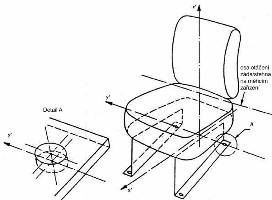
Obrázek 12 — Stanovení tří vztažných os pro SIP
