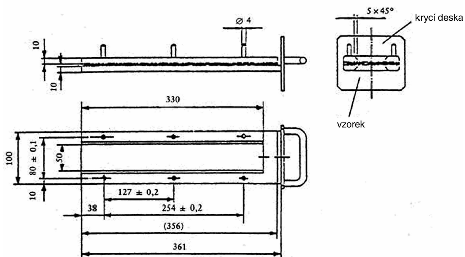
Obrázek 18 — Příklad držáku vzorků
