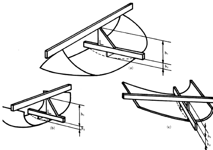
Obrázek 1 — Stanovení výšky h segmentu
