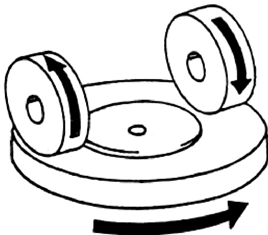
Obrázek 4 — Nákres principu přístroje pro odírání
