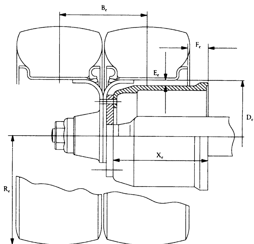
Obrázek 1 Řez sestavou nápravy
