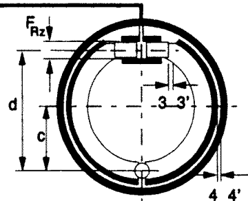
bubnová brzda
