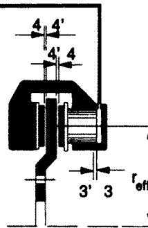
kotoučová brzda
