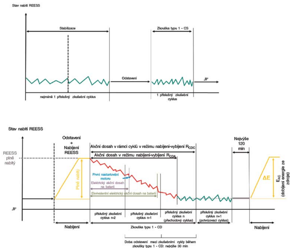
Vozidla OVC-HEV, zkouška typu 1 v režimu nabíjení-vybíjení s následnou zkouškou typu 1 v režimu nabíjení-udržování
