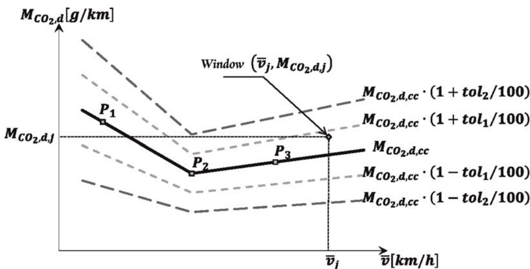
Charakteristická křivka CO 2 vozidla
