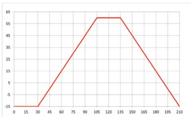
Obrázek VI.3 Cyklus regulace teploty
