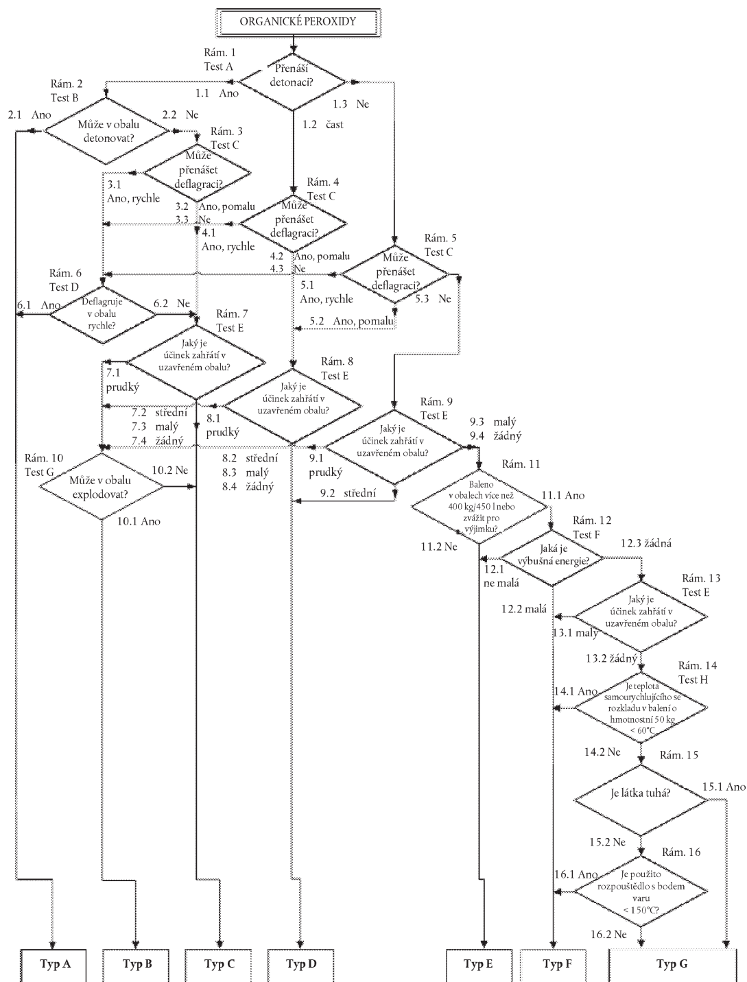
Obrázek 2.15.1 Organické peroxididy
