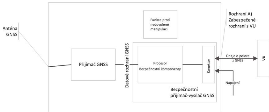
Obrázek 4 Schéma vnějšího zařízení GNSS
