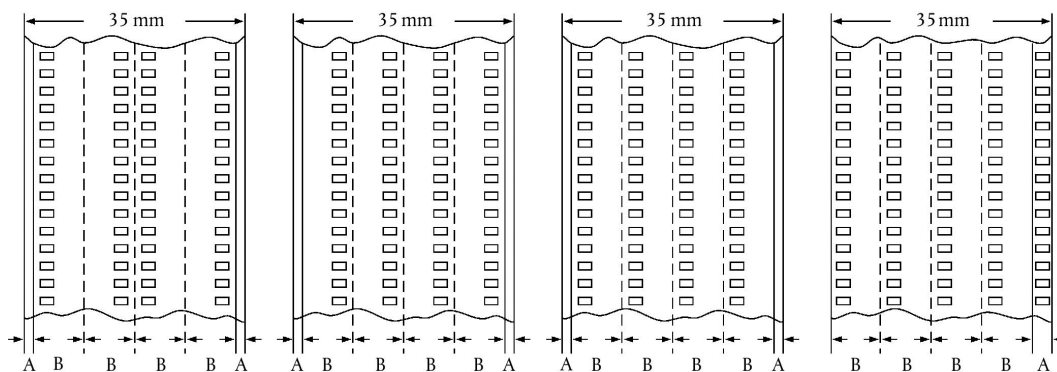
Видове филми с няколко ленти за образ
