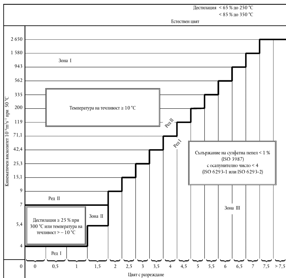
Характеристики на тежките горива (fuel oils)
