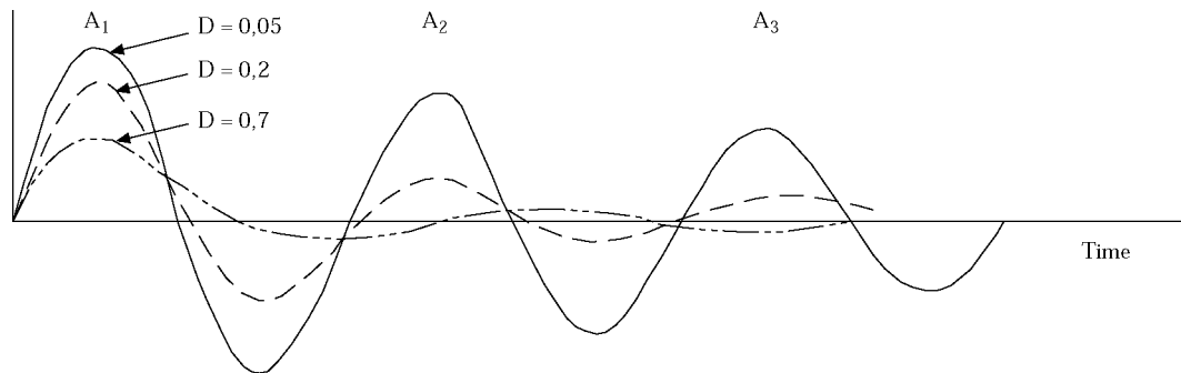
Приглушена синусоида при кратковременно свободно трептене
