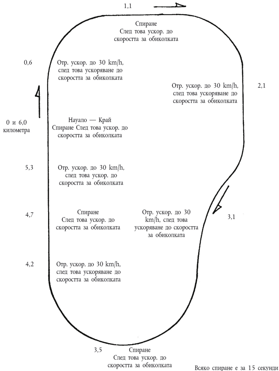
График за движение в рамките на подподцикъл от изпитването АМА
