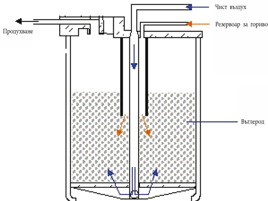
Диаграма на газовия поток във въгленовия филтър и отвори
