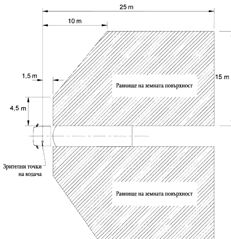
Фигура 9: Зрително поле при широкоъгълно огледало за обратно виждане от клас IV
