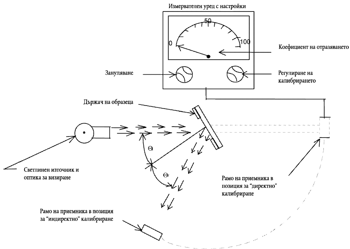
Фигура 4: Обобщен рефлектомер, показващ експериментални схеми за двата метода за калибриране
