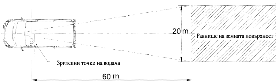
Фигура 6: Зрително поле при огледала от клас I
