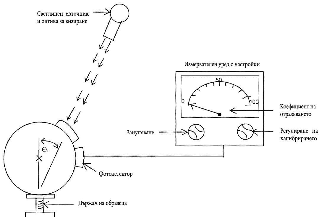
Фигура 5: Обобщен рефлектомер, включващ в приемника нитегрираща сфера
