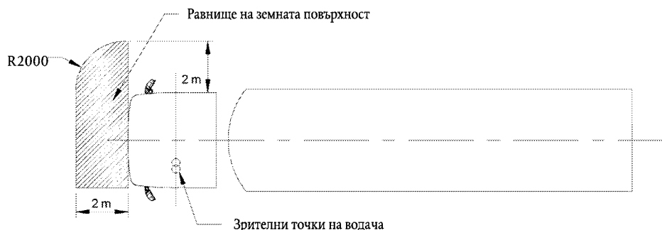
Фигура 11: Зрително поле при огледало от клас VI
