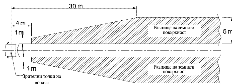
Фигура 7: Зрително поле при огледала от клас II
