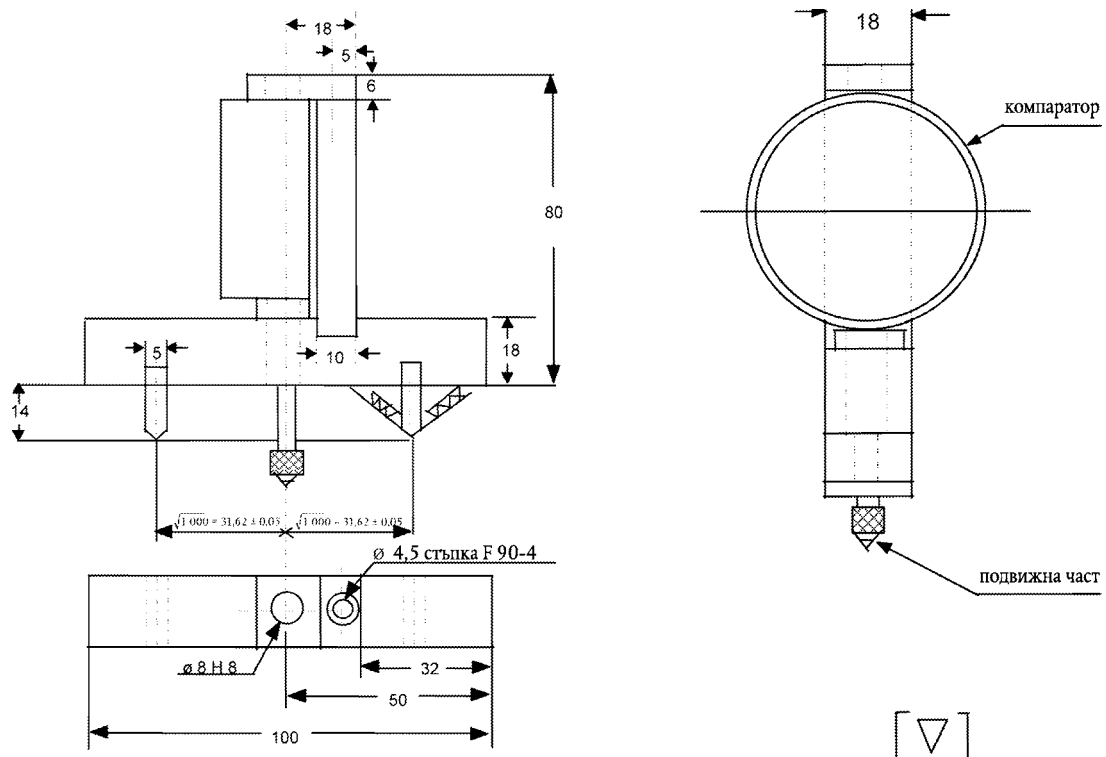
Фигура 3: Сферометър
