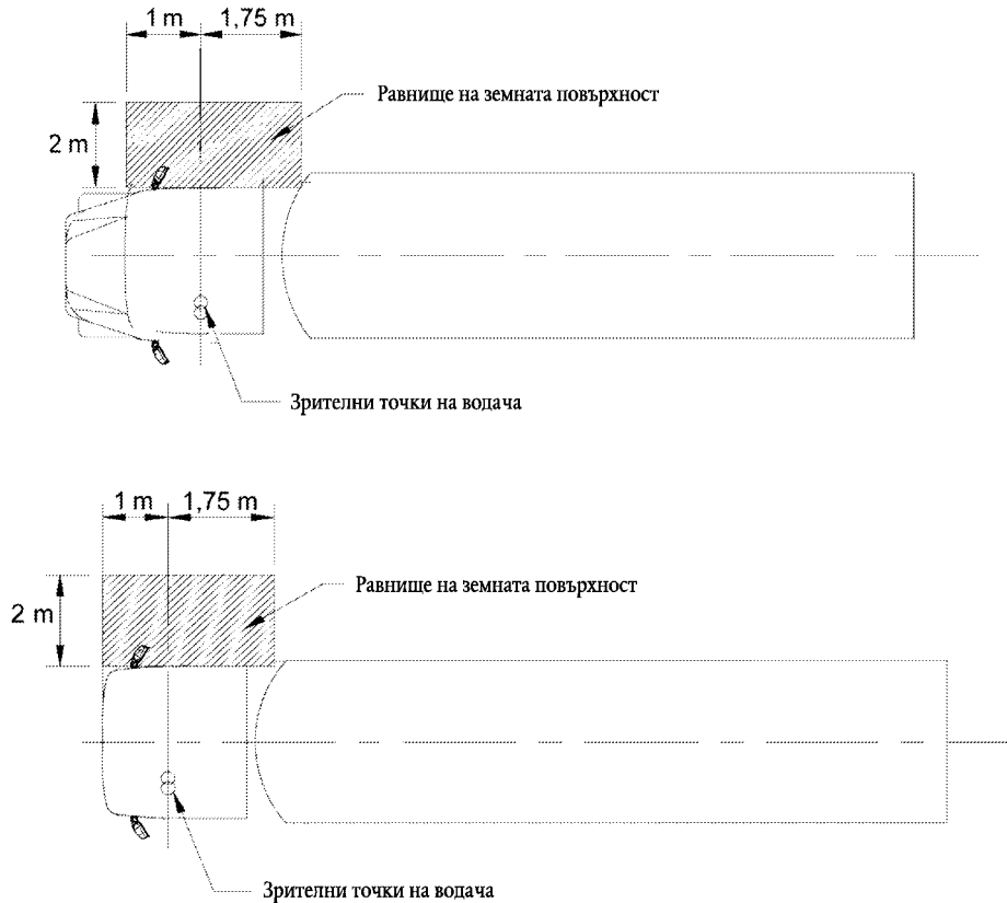
Фигура 10а и 10б: Зрително поле при широкоъгълно огледало за обратно виждане „в непосредствена близост“ (клас V)
