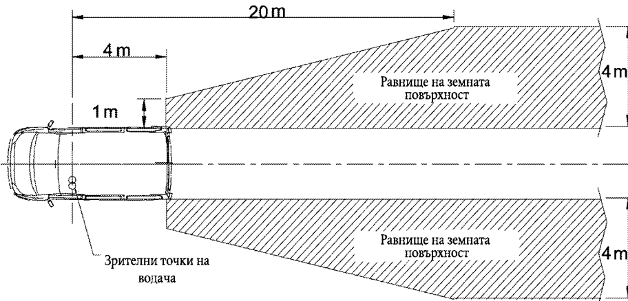
Фигура 8: Полезрение при огледала от клас III
