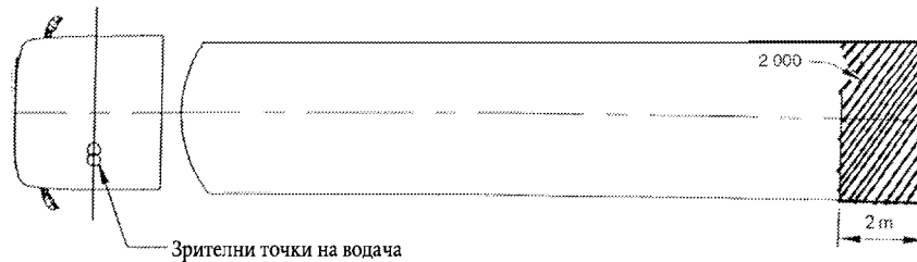
Фигура 12: Зрително поле при задно разположени устройства за непряко виждане
