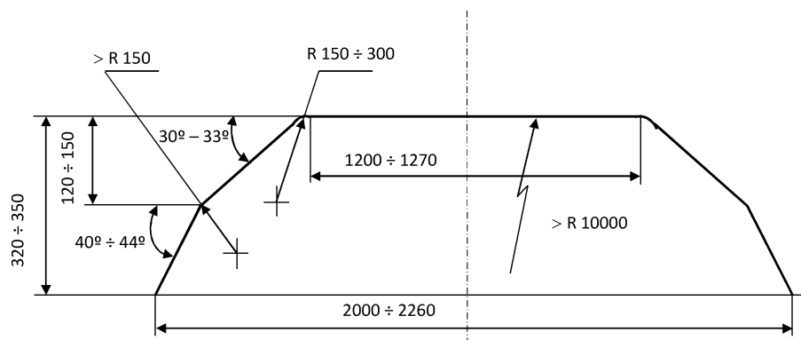
Фиг. Конфигурация и размери на контактните плъзгачи
