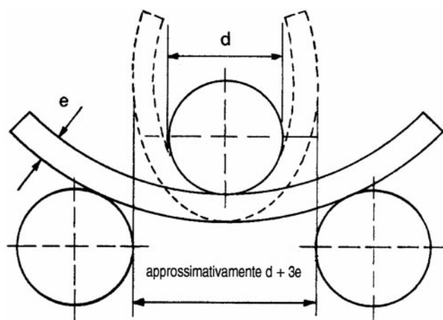
Schema della prova di piegamento
