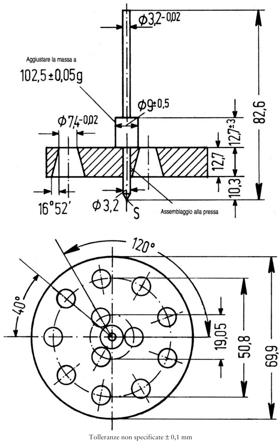
Figura 3 — Penetrometro
