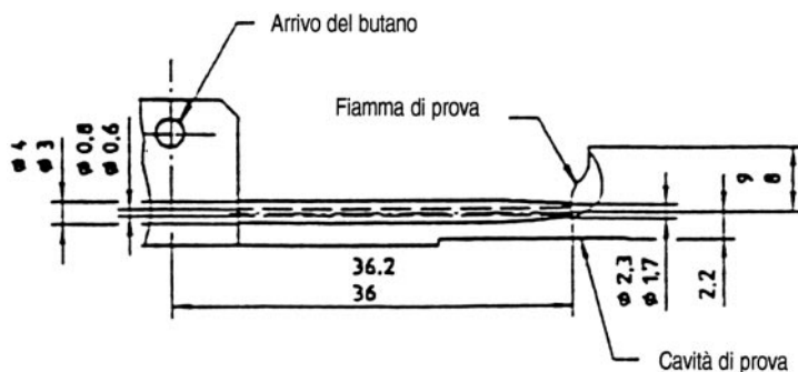
Figura 2 — Becco a gas e fiamma di prova
