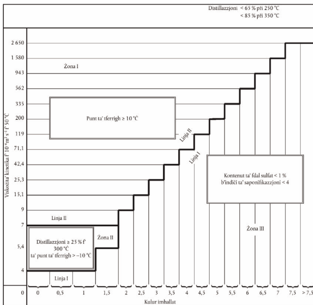
Karatteristiċi ta' żjut karburanti
