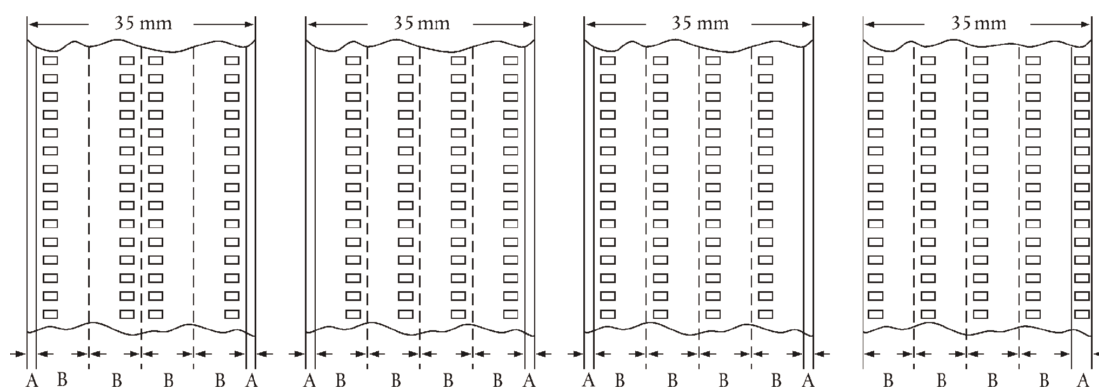
Τύποι φιλμ με πολλές σειρές εικόνων
