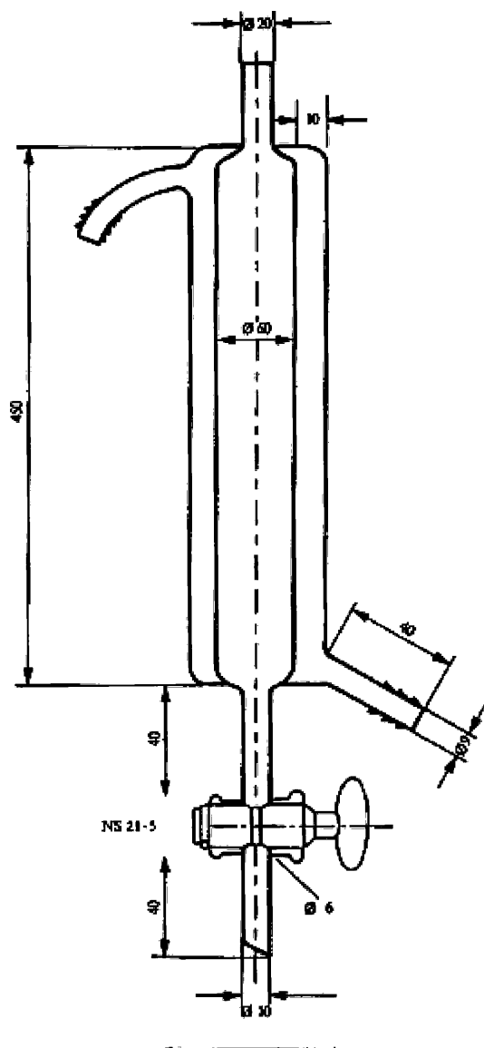
Rysunek 4 Kolumna wymiennika ciepła (wymiary w milimetrach)
