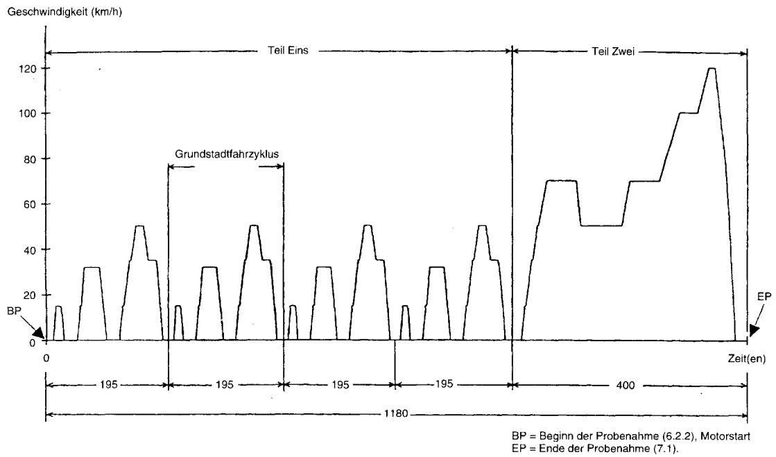
Abbildung III.1.1 Fahrzyklus für die Prüfung Typ I
