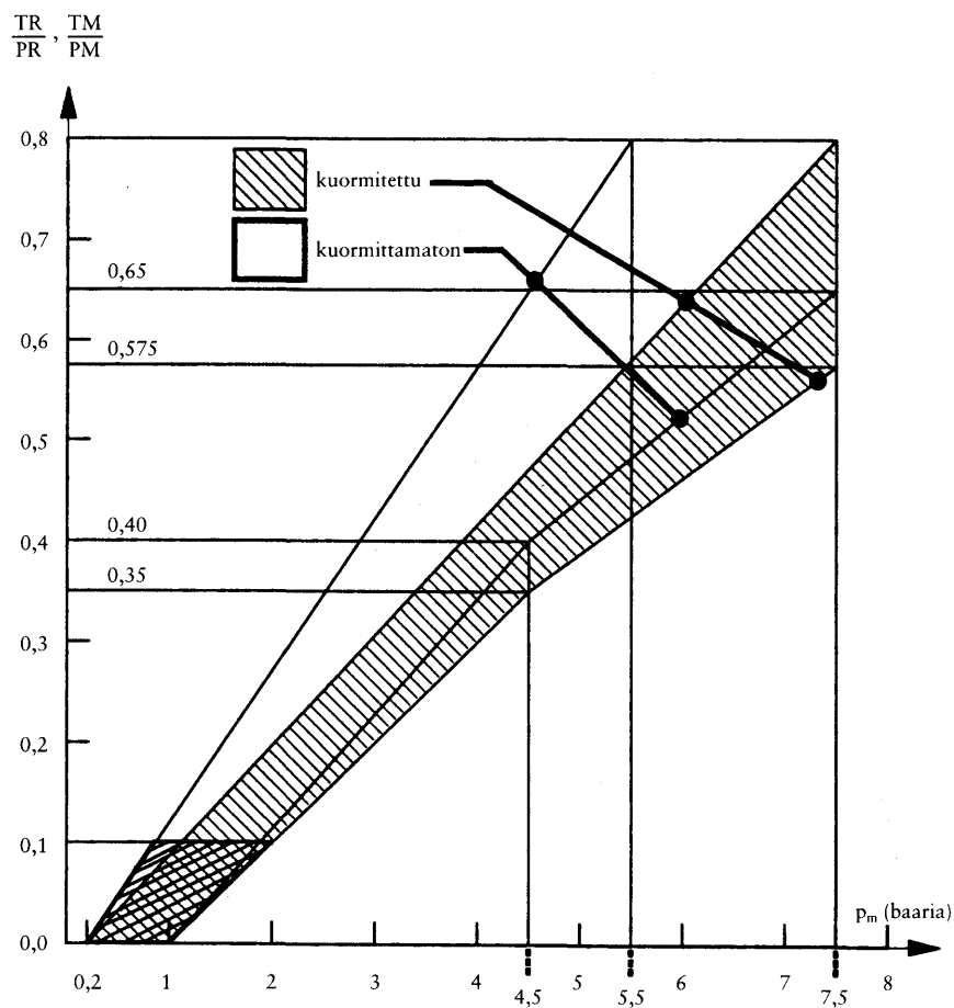
Kaavio 2 Vetoautot ja perävaunut (ks. 3.1.4 ja 5 kohta)
