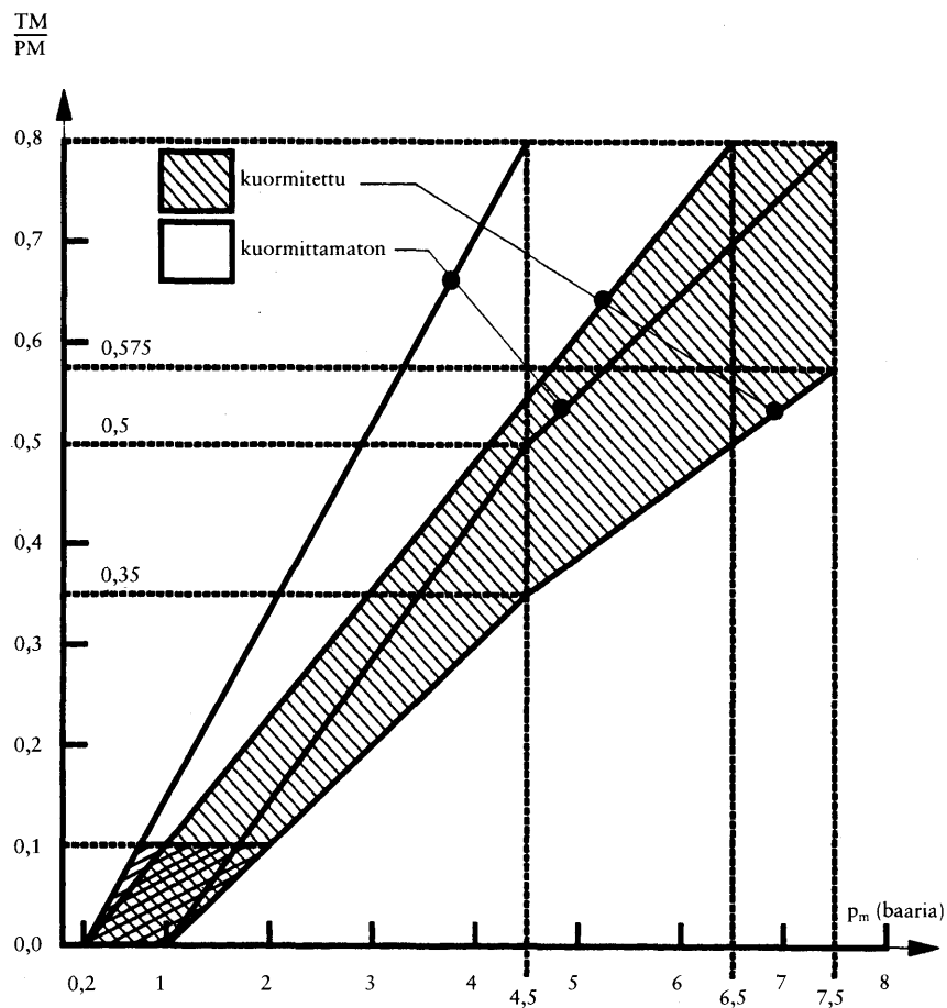
Kaavio 3 Puoliperävaunujen vetoautot (ks. 3.1.5 kohta)
