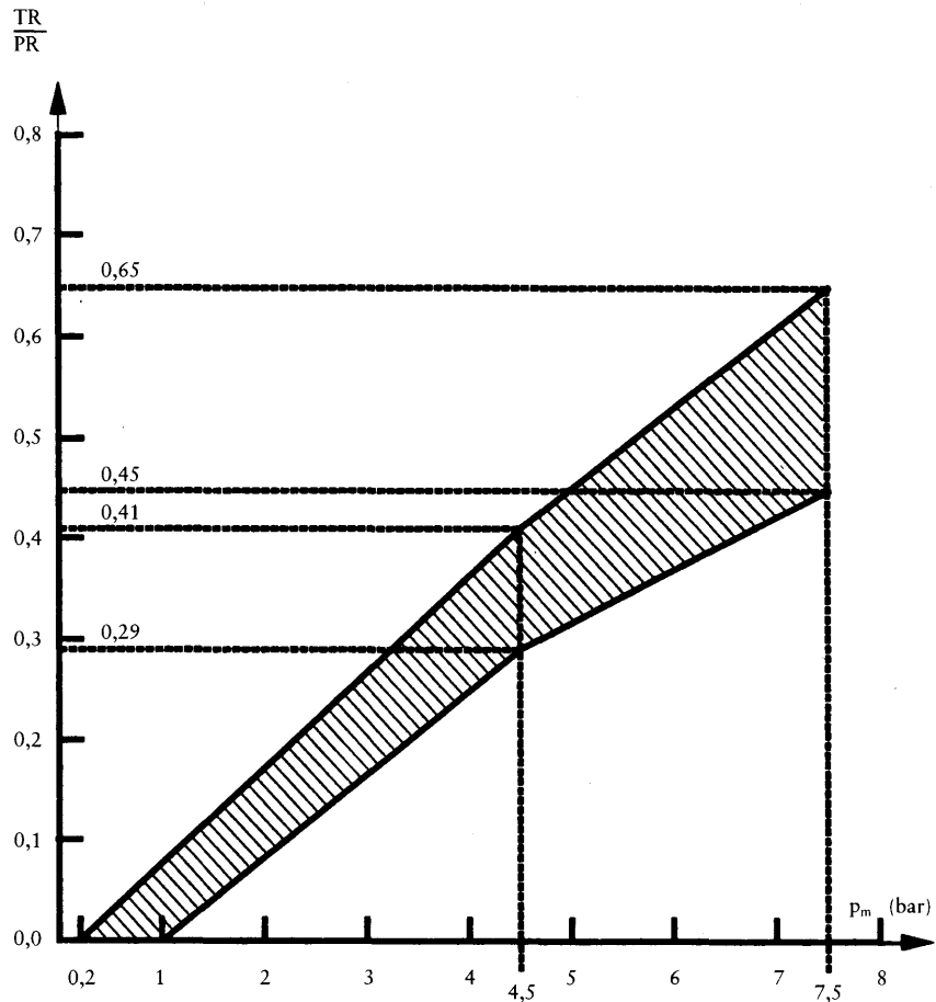
Kaavio 4A Puoliperävaunut (ks. 4 kohta)
