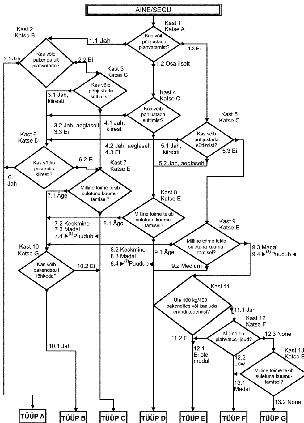
Joonis 2.15.1 Orgaanilised peroksiidid
