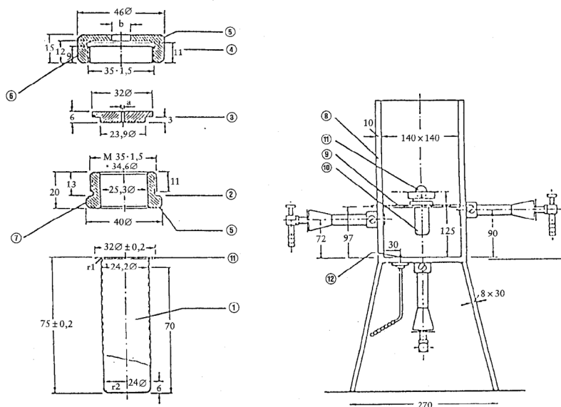
1.a att. Tērauda caurule ar piederumiem
