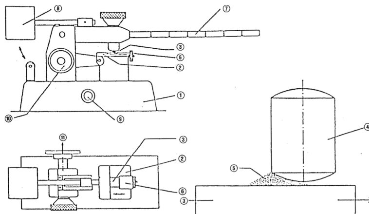
5.a att. Berzes aparāts; pretskats un augšskats
