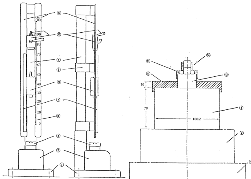
4.a att. Krītošais āmurs, priekšskats un sānskats, kopskats
