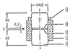
4.d att. Triecienierīce šķidru vielu testēšanai
