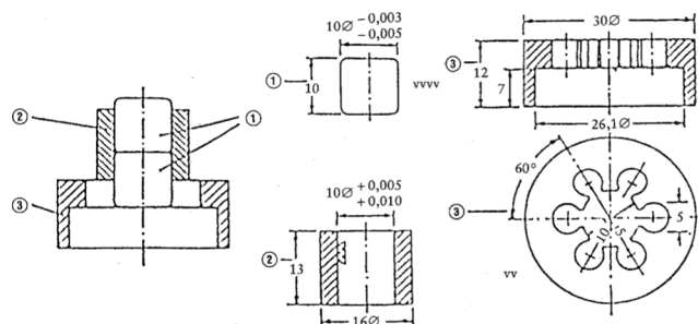
4.c att. Triecienierīce pulverveida vai pastveida vielu testēšanai
