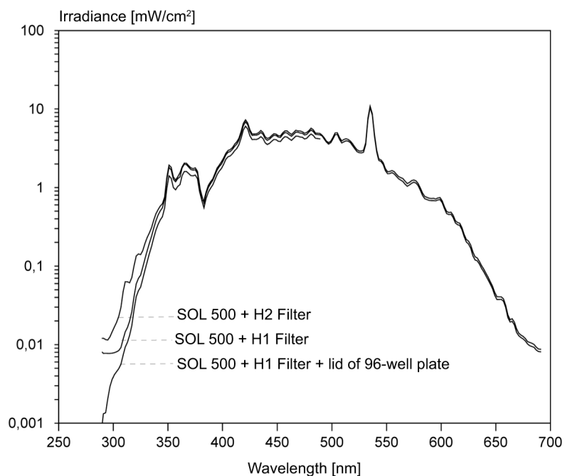
Saules gaismas imitatora filtrēta starojuma spektrālās jaudas sadalījums
