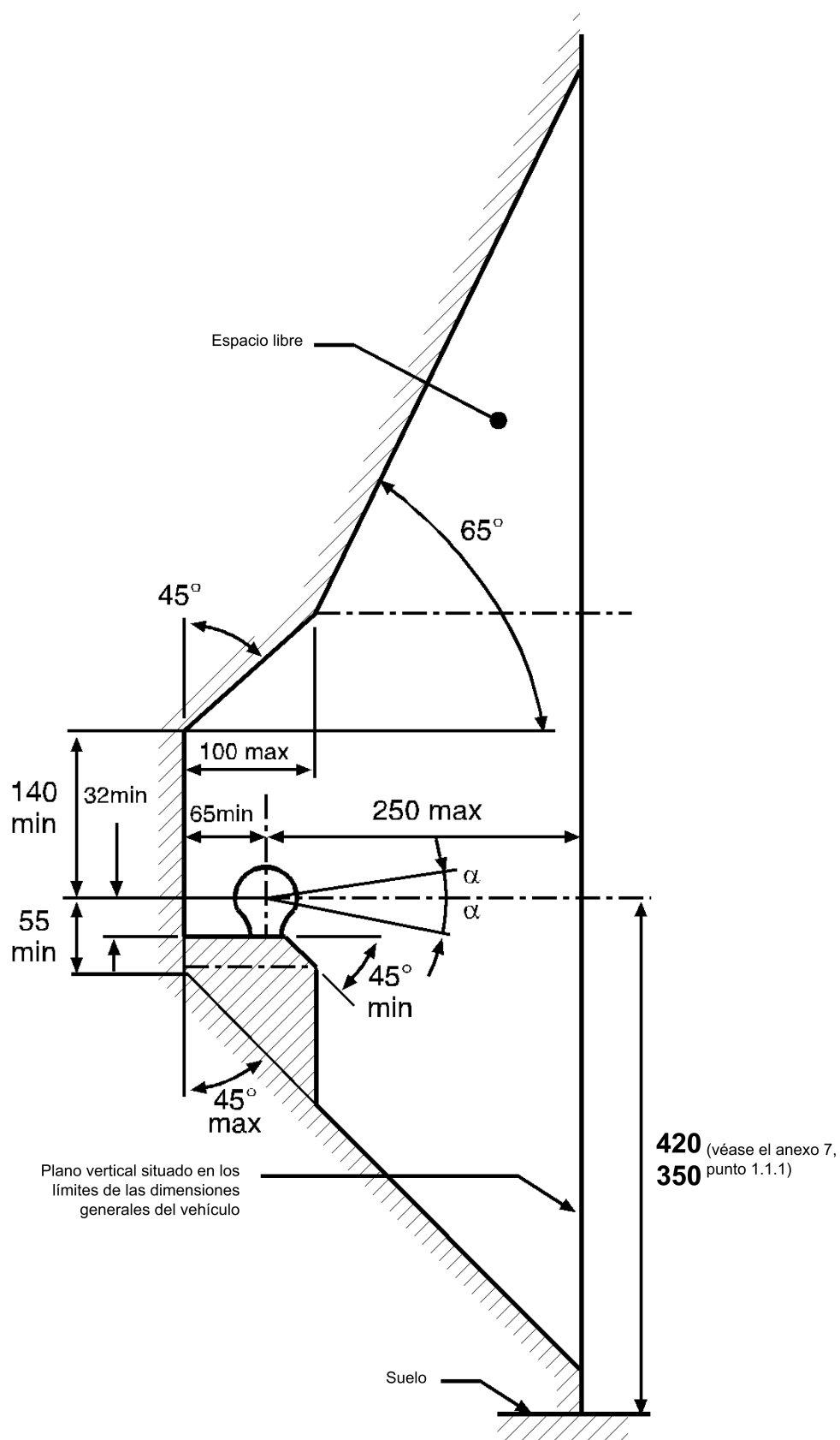
Figura 25a — Espacio libre y altura del acoplamiento de bola; vista lateral
