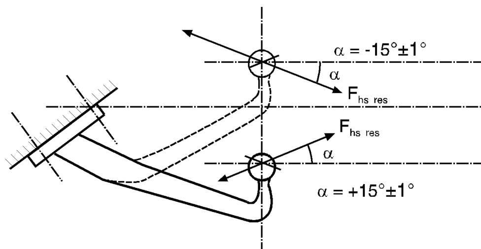
Figura 21 — Ángulos de aplicación de la fuerza de ensayo
