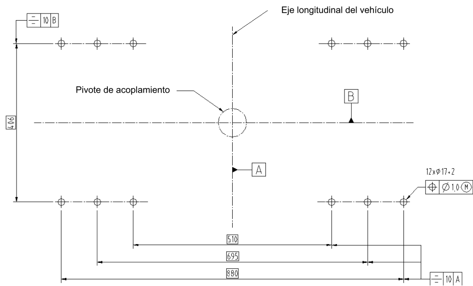
Figura 16a — Tolerancia de los orificios de montaje para placas de soporte de Clase J de acoplamientos de quinta rueda (véase el punto 9.1 del presente anexo)
