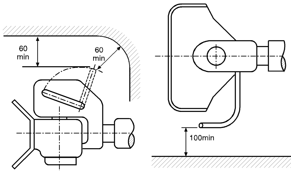
Figura 26 — Espacio libre para la palanca de mano
