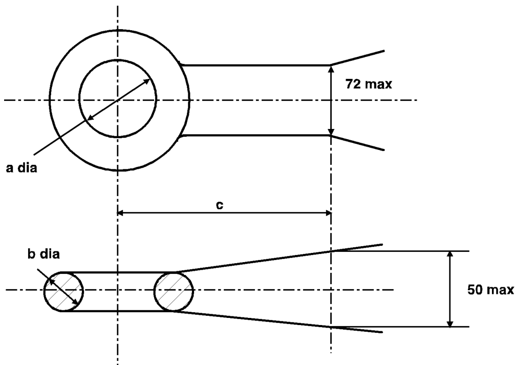
Figura 14 — Dimensiones de los anillos de remolque toroidales de Clase L (véase el cuadro 8)
