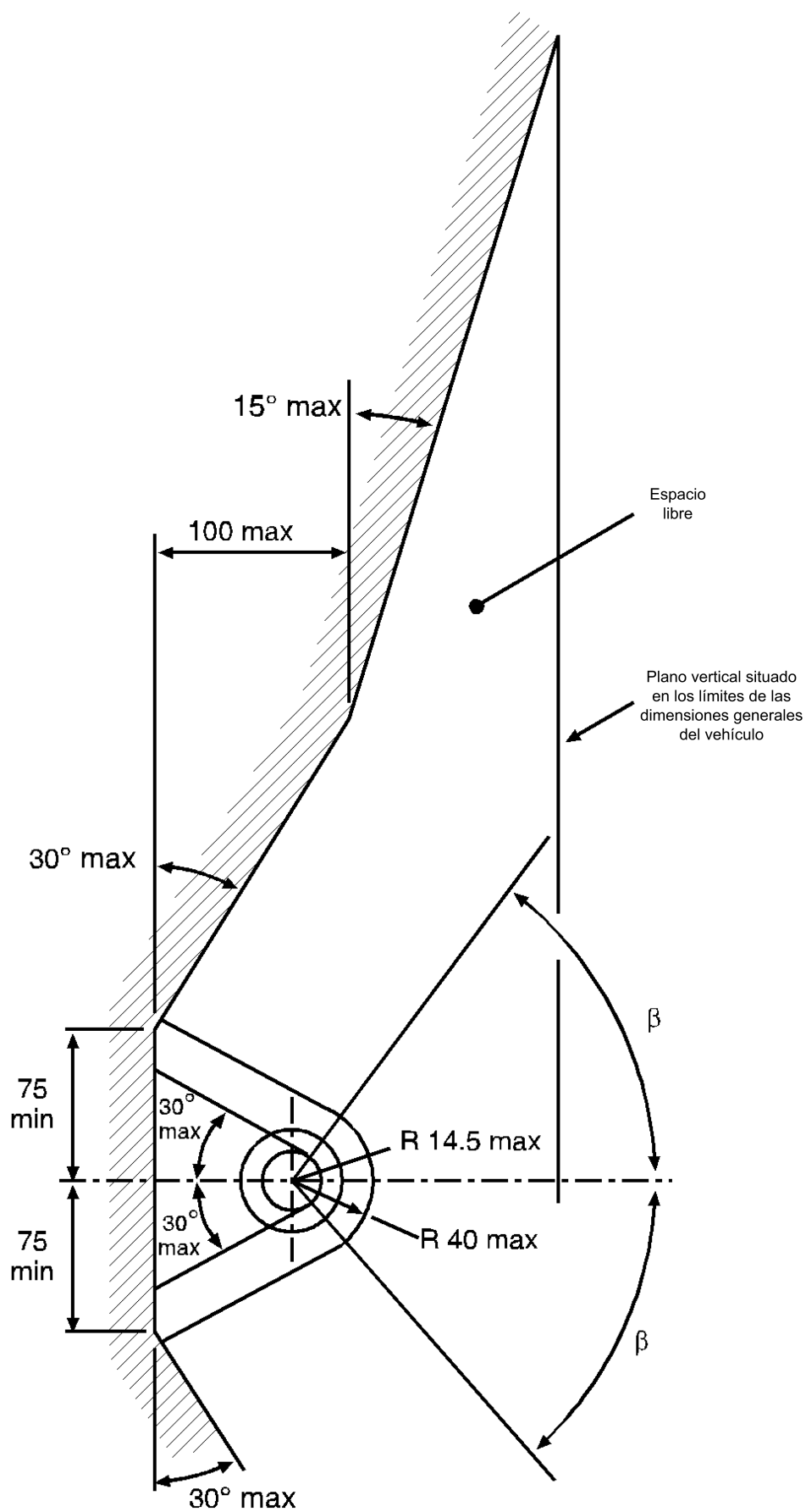
Figura 25b — Espacio libre del acoplamiento de bola; vista general
