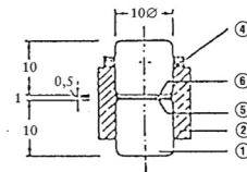
Figura 4d Dispositivo para o ensaio de choque de substâncias líquidas
