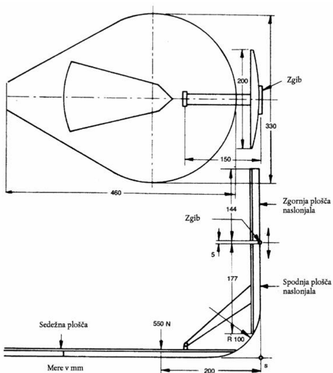
Slika 7 Naprava za določanje referenčne točke sedeža
