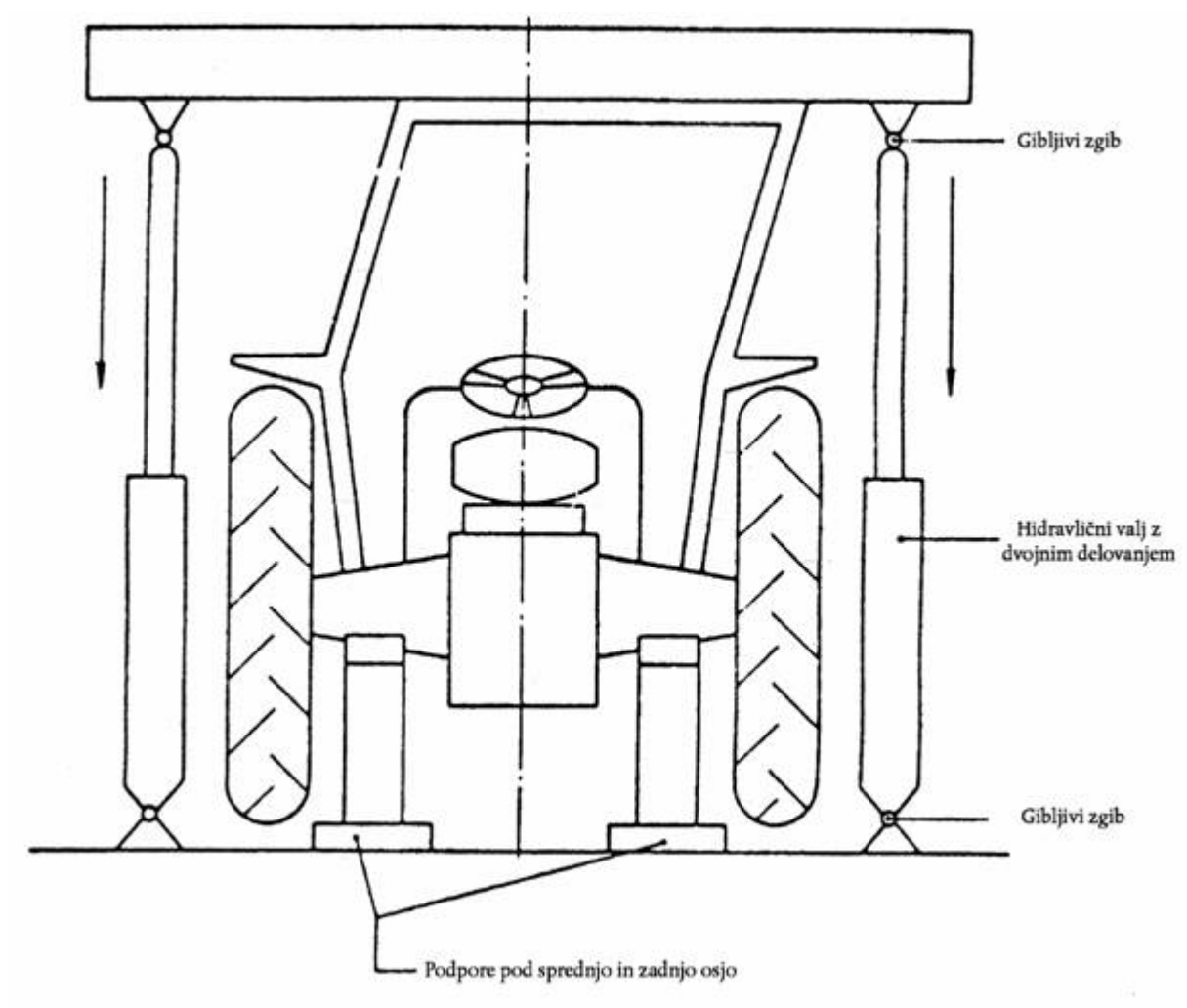
Slika 3 Primer naprave za tlačni preskus
