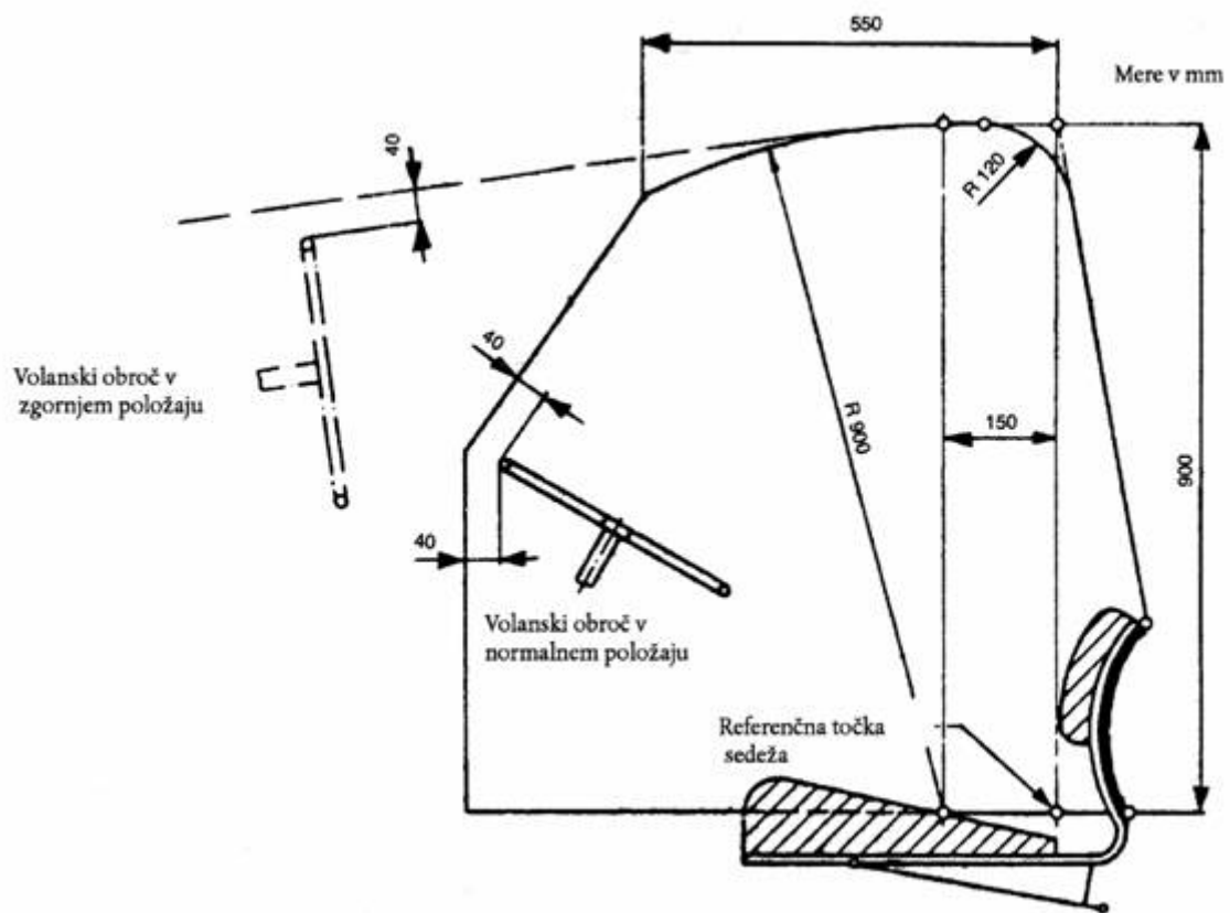
Slika 6a Stranski pogled na varen prostor
