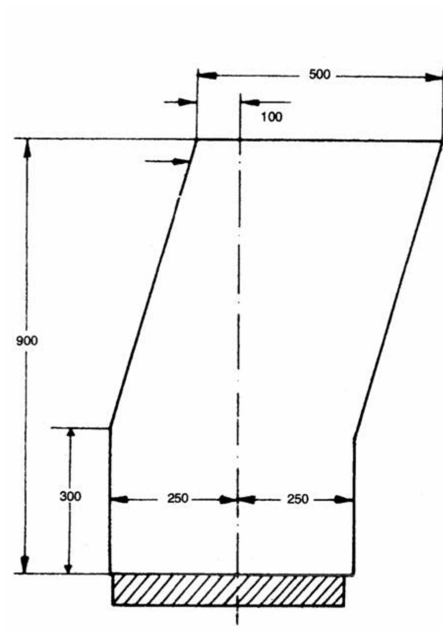
Slika 6b Pogled od spredaj/zadaj na varen prostor
