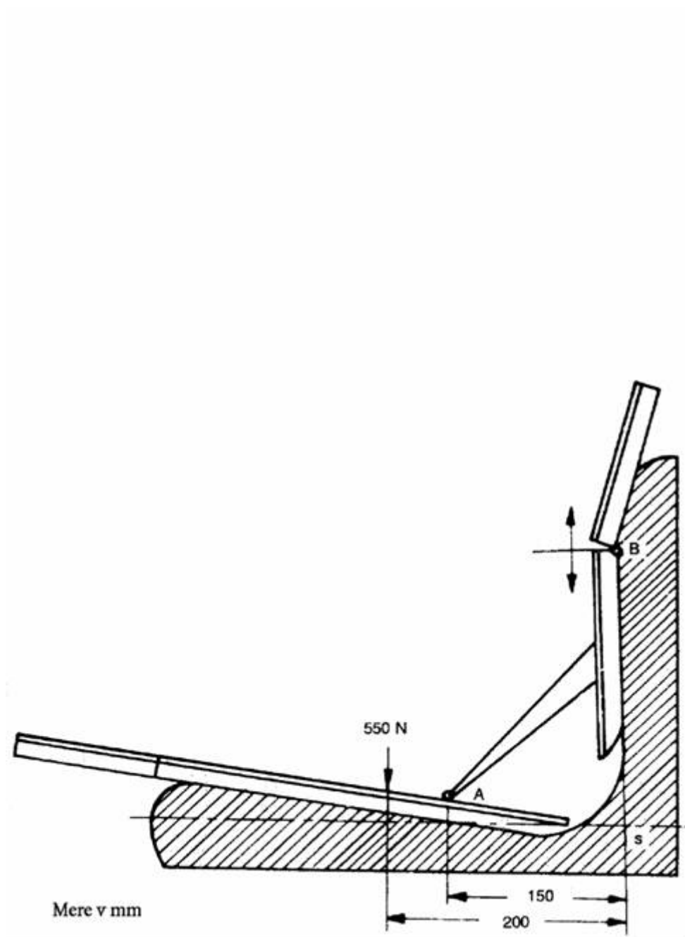
Slika 8 Postopek določanja referenčne točke sedeža
