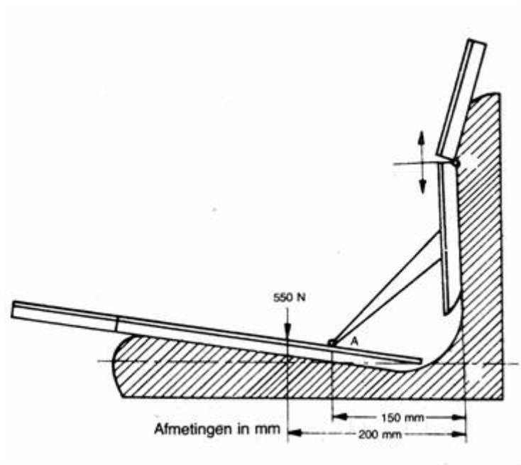
Figuur 8 Bepaling van het referentiepunt van de zitplaats
