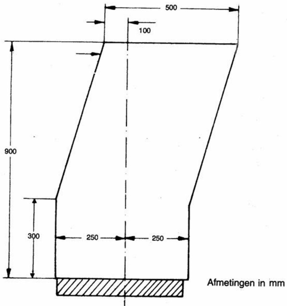
Figuur 6b Voor/achteraanzicht van de vrije zone
