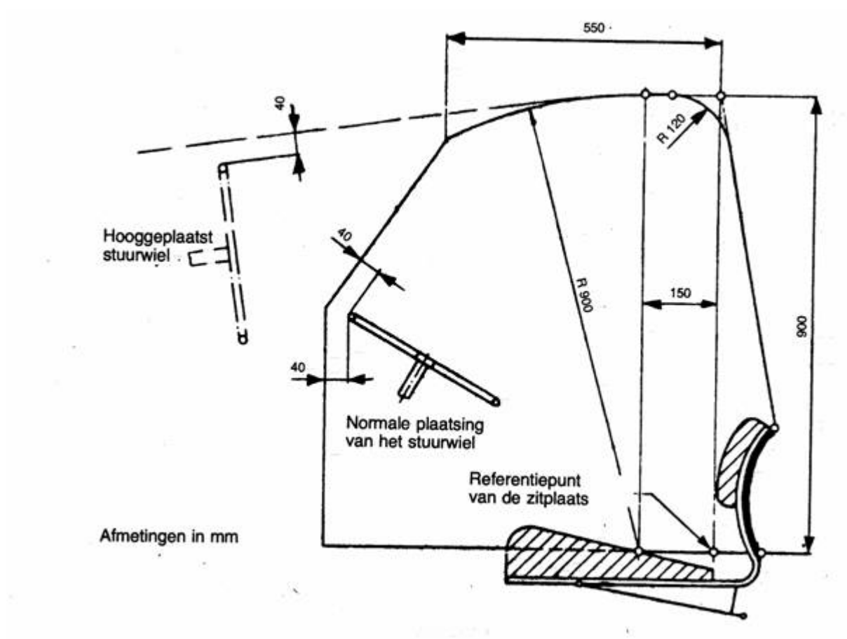
Figuur 6a Zijaanzicht van de vrije zone
