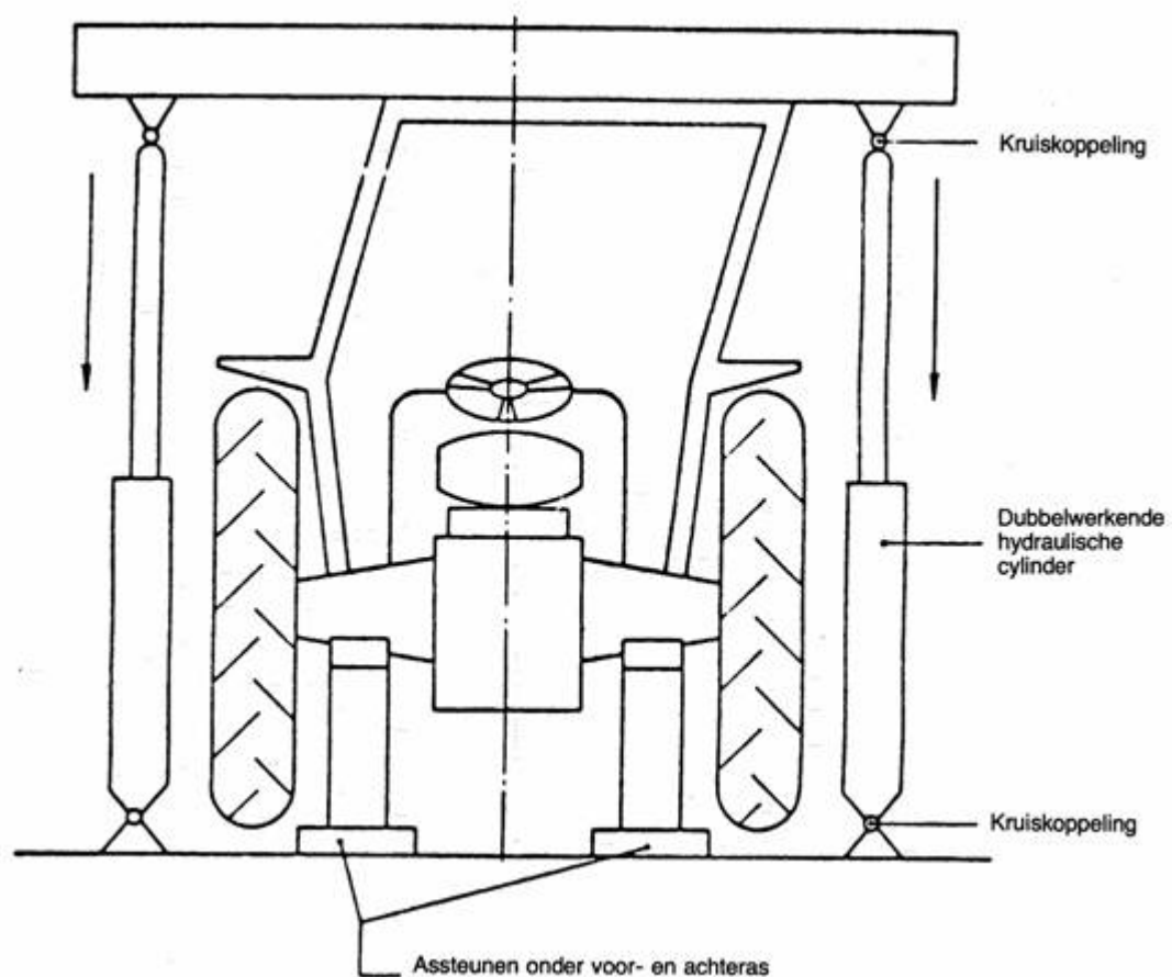
Figuur 3 Voorbeeld voor een opstelling voor een drukproef
