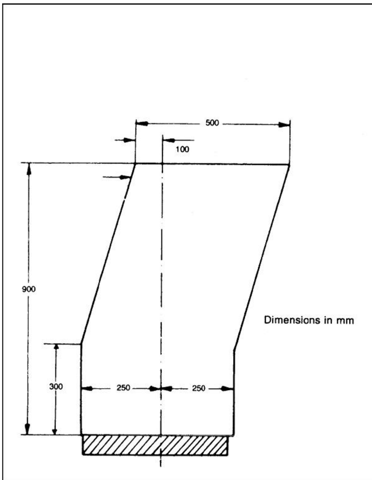
Figura 6b: Dehra minn quddiem/wara taż-żona ta' spazju
