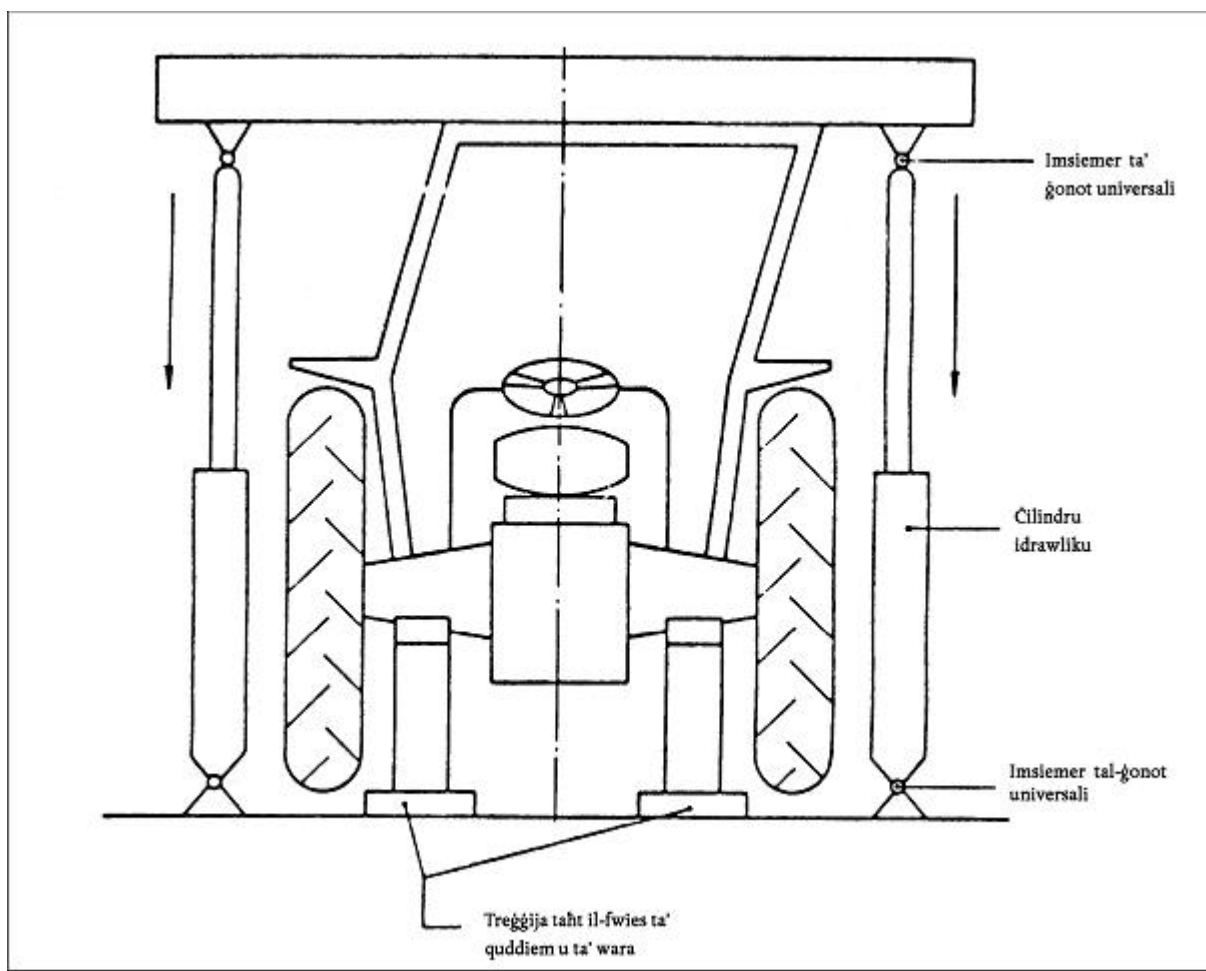
Figura 3: Eżempju ta' arrangament għal kontroll ta' tghaffiġ
